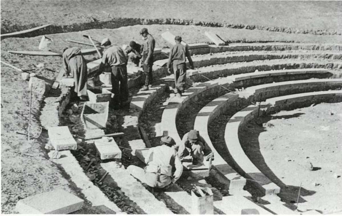
52- Hasanođlan Köy Enstitüsü açık hava tiyatrosu inřaati (Proje: Y.Mimar Mualla Eyubođlu)
